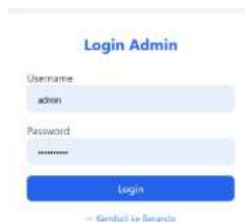
Gambar 3. Tampilan Login
