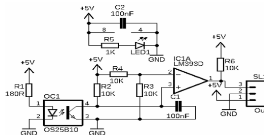
Gambar 2.2. Rangkaian Optocoupler
